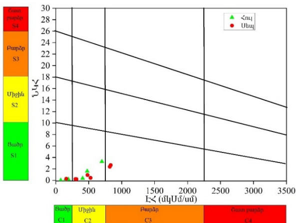
Գծանկար 3. 2017 թ. Ողջի գետի ջրհավաք ավազանի գետաջրերի ոռոգելի հատկությունները՝ ԱՄՆ աղիության լաբորատորիայի (USSL) գծապատկերի համաձայն
