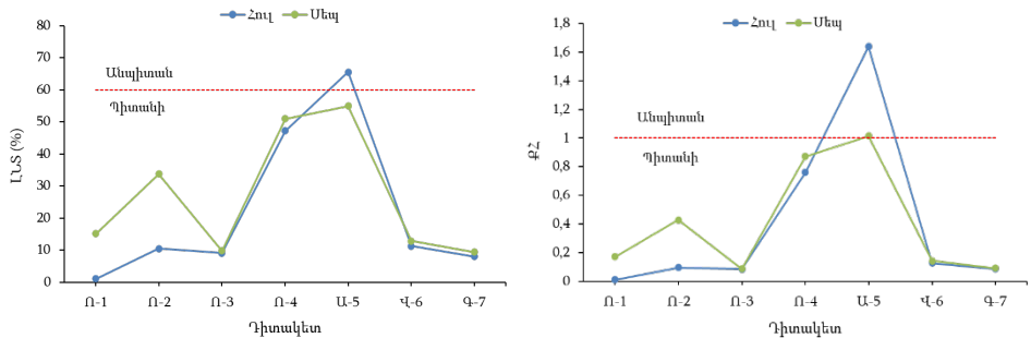
Փճանկար 4. 2017 թ. Ողջի գետի ջրի վաղաք ավազանի գետաջրերում ԼՆՏ և ՔՀ արժեքները՝ ոռոգման նպատակով ջրօգտագործման պիտանելիության շեմի համեմատությամբ
