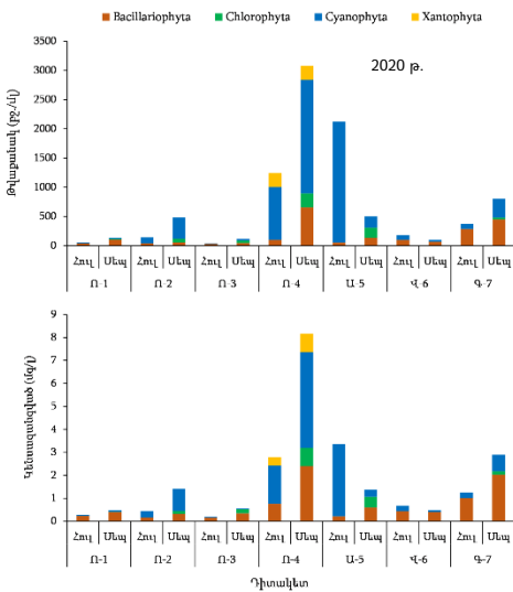
Փծանկար 8. Ողջի գետի ջրիավաք ավազանի գետաէկոհամակարգերի ֆիտոպլանկտոնային համակեցության քանակական ու որակական ցուցանիշների տարածաժամանակային բաշխվածությունը
