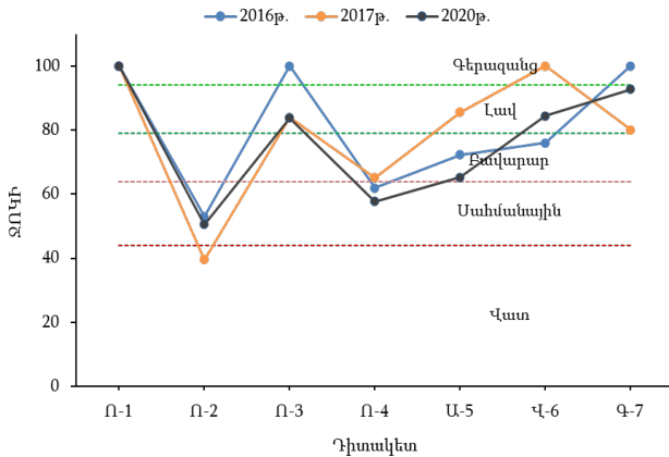
Գծանկար 7. Ողջի գետի ջրհավաք ավազանի գետաջրերում ՋՈԿԻ արժեքները՝ ջրի որակի դասակարգման համեմատությամբ
