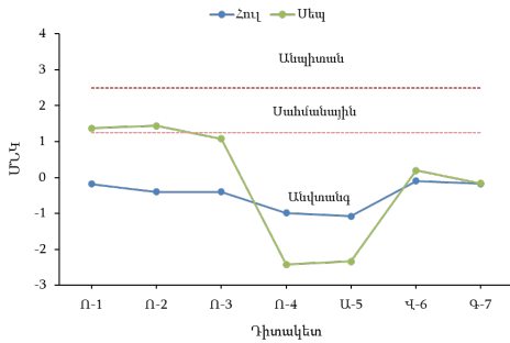
Գծանկար 5. 2017 թ. Ողջի գետի ջրհավաք ավազանի գետաջրերում ՄՆ_4 և ՄՆ_2 արժեքները՝ ոռոգման նպատակով ջրօգտագործման պիտանելիության դասակարգման համեմատությամբ
