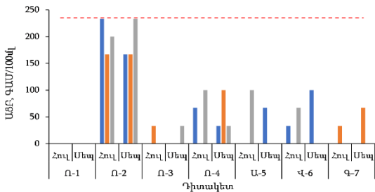
Փձանկար 6. Ողջի գետի ջրիավաք ավազանի գետաջրերում ԸԿԲ, ՖԿԲ ու ԱՑԲ կոնցենտրացիաները՝ ոռոգման ու ռեկրեացիոն նպատակով ջրօգտագործման նորմերի համեմատությամբ
