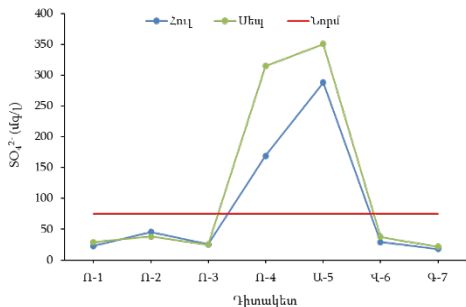
Փձանկար 2. 2017 թ. Ողջի գետի ջրավաք ավազանի գետաջրերում K^+ , Na^+ ու SO_4^{2-} իոնների կոնցենտրացիաները՝ գետաջրերի որակի երկրորդ դասի նորմի համեմատությամբ
