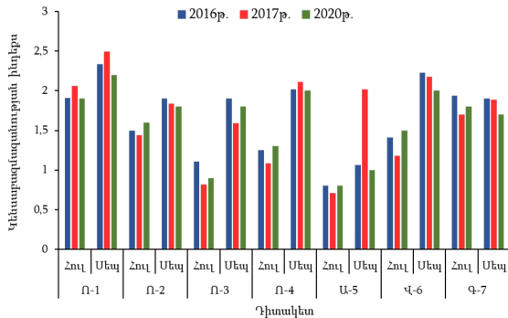
Գծանկար 9. Ողջի գետի ջրհավաք ավազանի գետաէկոհամակարգերի ֆիտոպլանկտոնային բազմազանության (Շաննոն-Վիների ցուցիչ) տարածաժամանակային փոփոխությունները
